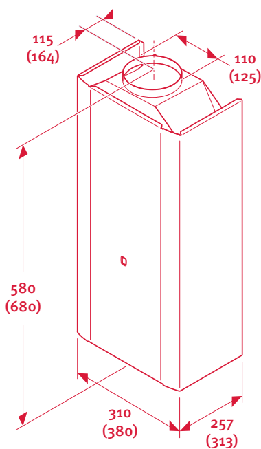
Připojovací rozměry průtokového ohřívače Panda 19 (24) POG E-B
