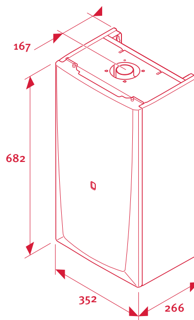
Připojovací rozměry průtokového ohřívače Panda 24 PTP
