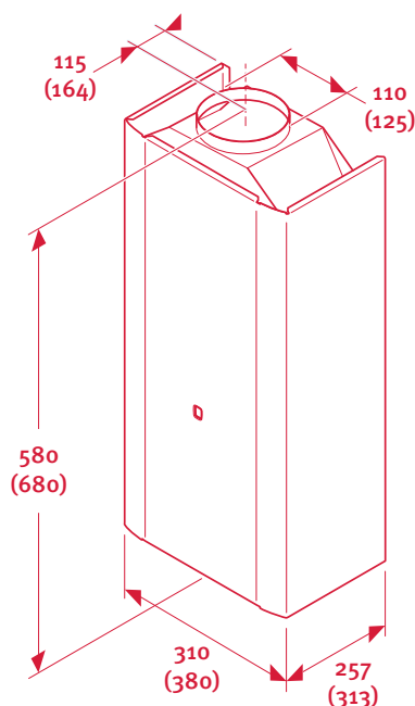
Připojovací rozměry průtokového ohřívače Panda 19 (24) POG E-B
