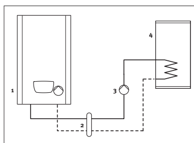
Hydraulické zapojení zásobníkového ohřívače
