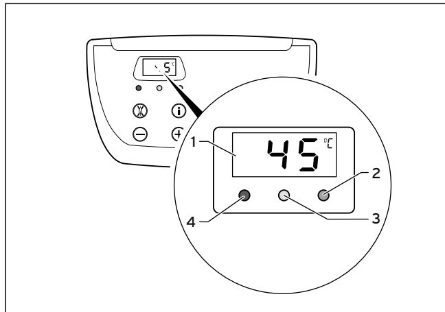
Obr. 6.2 Indikační svítilny
