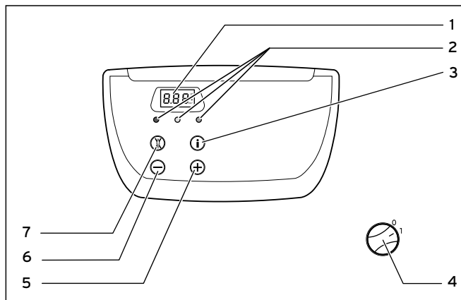
Obr. 6.1 Ovládací prvky
